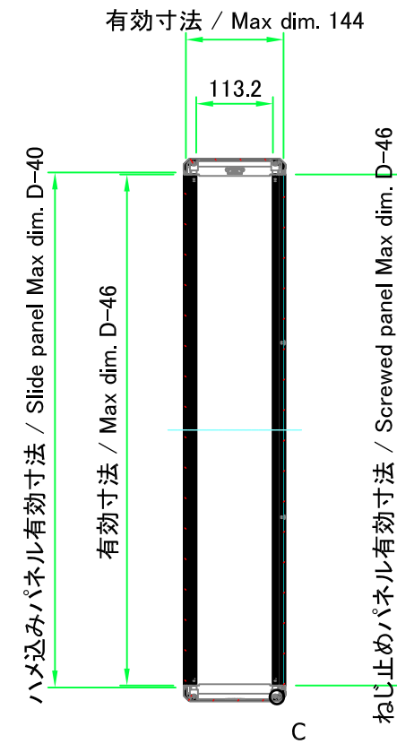
B-B ( 1 : 10 )
