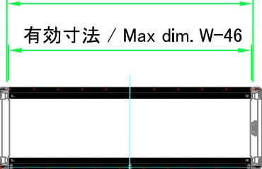
A-A ( 1 : 10 )
